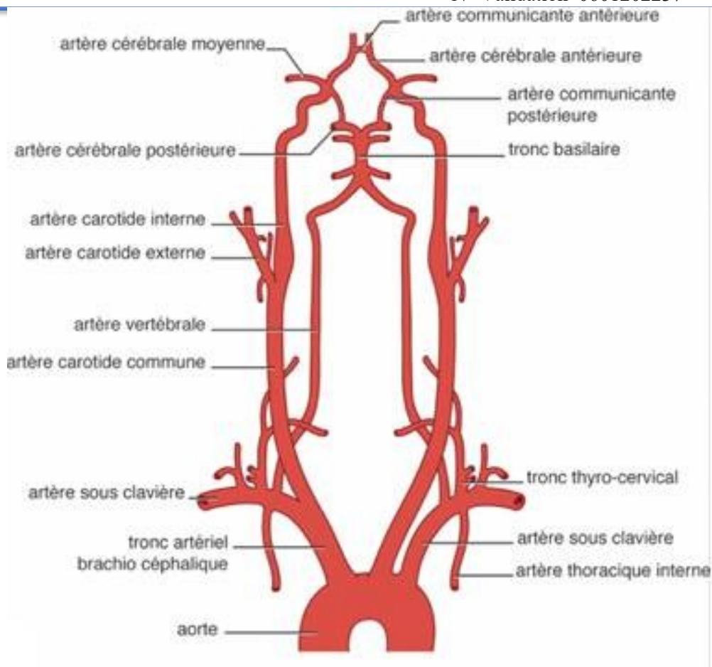
Figure 1 : Artères cervico-encéphaliques
